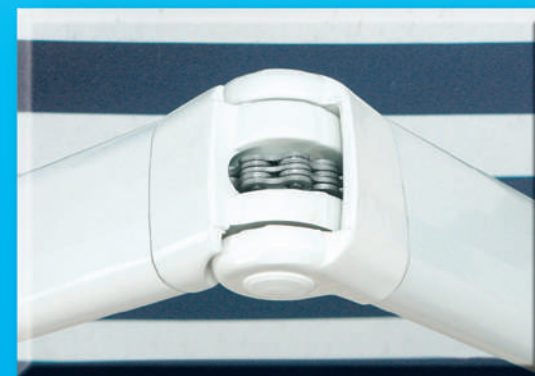
Gelenkarm mit extra starker Flyer-Kette
